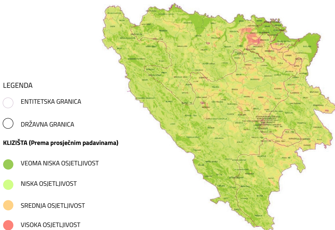
Slika 5. Distribucija zona podložnih na kliženje u Bosni i Hercegovini
